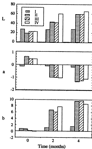
圖三：柚子皮蜜餞製品貯藏期間之顏色變化
