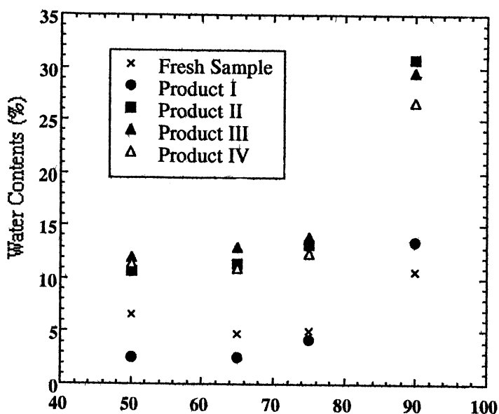
圖一：柚子皮與其蜜餞製品在25°C下之吸濕曲線
